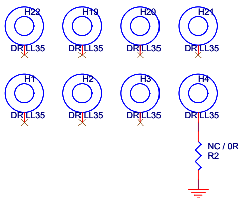
底板固定孔
