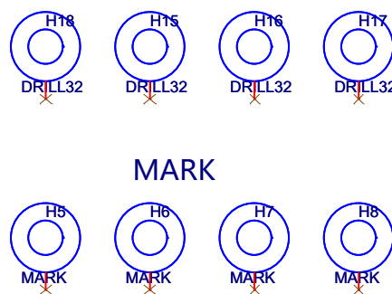
Pi固定孔
